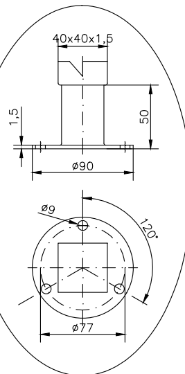
PARTICOLARE PIEDE FOOT DETAIL
